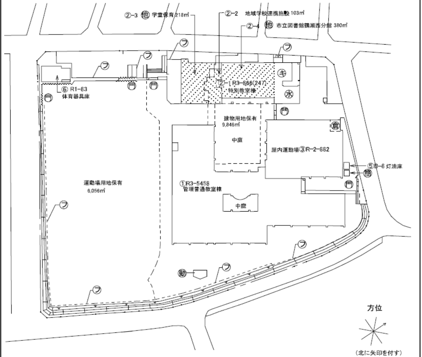
敷地・建物全体図
