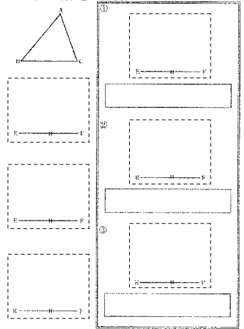
P93 三角形の合同条件 △ABCと合同な三角形を書けよう。
