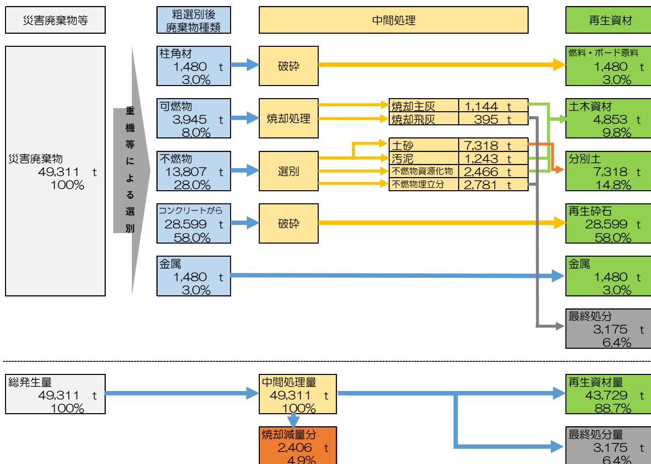
図3-2 災害廃棄物処理フロー（地震）
